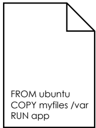
Dockerfile
